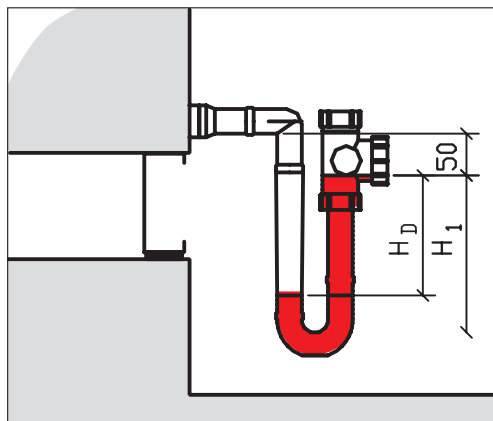
Überdruck im Gerät
