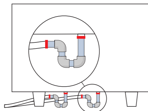
Abb. 4.5.3.1 Installation Kondensatablauf
