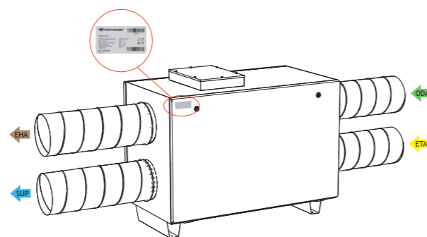
Abb. 1.4 Platzierung technischer Aufkleber und Luftkanalanschluss GS-H-70 (linke Version)
