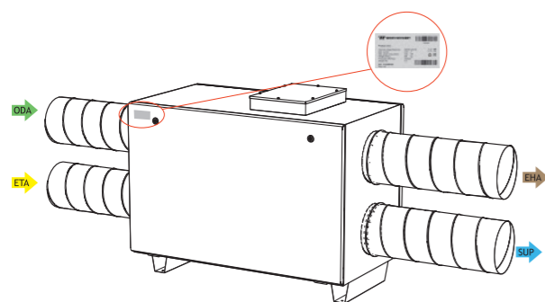
Abb. 1.3 Platzierung technischer Aufkleber und Luftkanalanschluss GS-H-70 (rechte Version)
